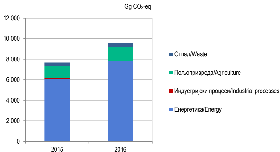
Графикон 1. Емисија директних гасова са ефектом стаклене баште (искључујући поноре), по секторима Graph 1. Direct greenhouse gas emissions (excluding sinks), by sectors
