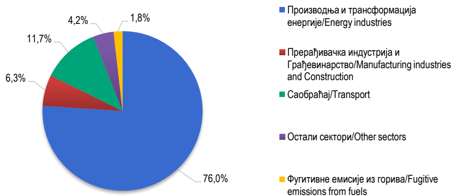
Графикон 2. Структура емисије гасова са ефектом стаклене баште из Енергетике, по подсекторима, 2016. Graph 2. Structure of the of greenhouse gas emissions from Energy, by subsectors, 2016
