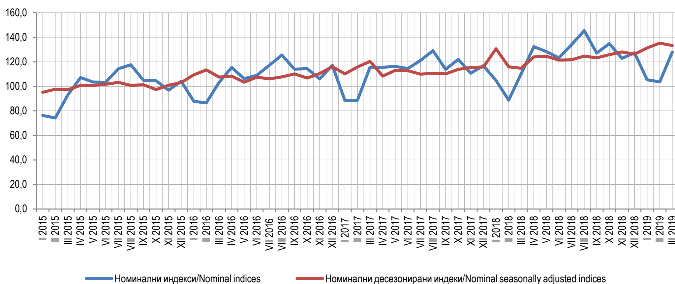
Графикон 1. Серија номиналних неприлагођених и десејонизираних индекса, 2015=100 Graph 1. Series of nominal non-adjusted and seasonally adjusted indices, 2015=100
