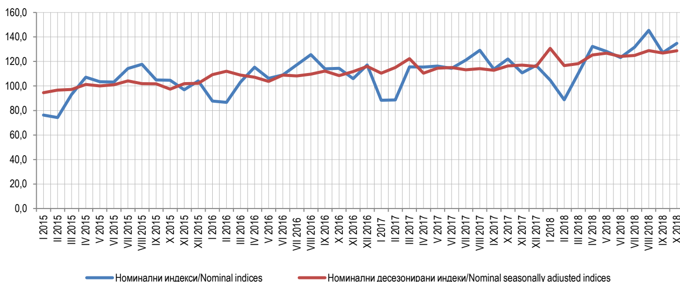
Графикон 1. Серија номиналних неприлагођених и десејонизираних индекса, 2015=100 Graph 1. Series of nominal non-adjusted and seasonally adjusted indices, 2015=100
