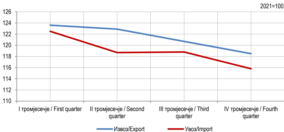
Графикон 1. Индекси извозних и увозних цијена, по тромјесечјима, 2023. (KM) Graph 1. Export and import price indices by quarter, 2023 (KM)
