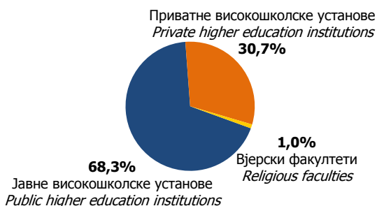
Графикон 2. Студенти према облику својине високошколске установе у школској 2010/2011. години Graphic 2. Enrolled students by type of ownership of higher education institution in the academic year 2010/2011
