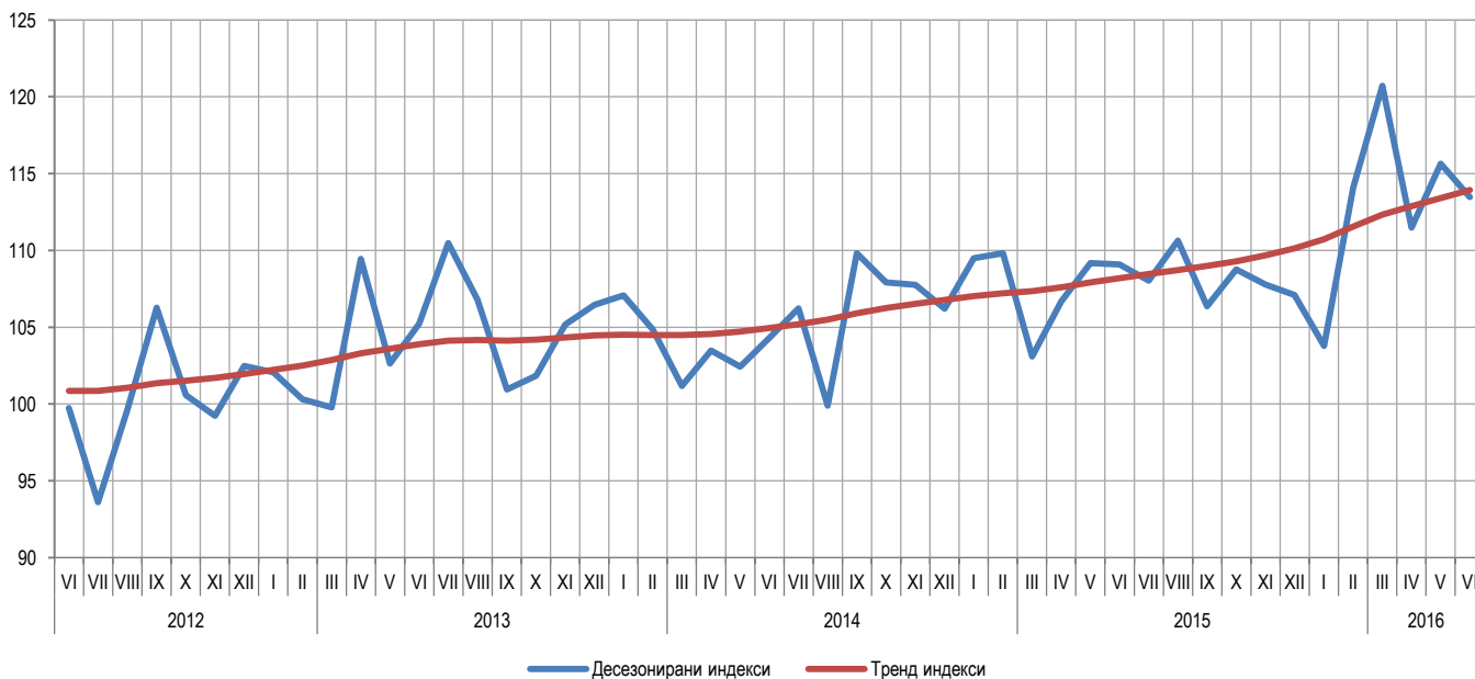
Графикон 1. Индекси индустријске производње, јун 2012 – јун 2016. (2010=100) Graph 1. Indices of industrial production, June 2012 – June 2016 (2010=100)
