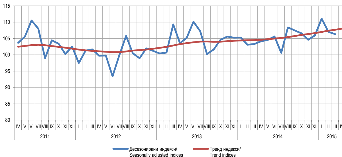
Графикон 1. Индекси индустријске производње, април 2011 – април 2015. (2010=100) Graph 1. Indices of industrial production, April 2011 – April 2015 (2010=100)
