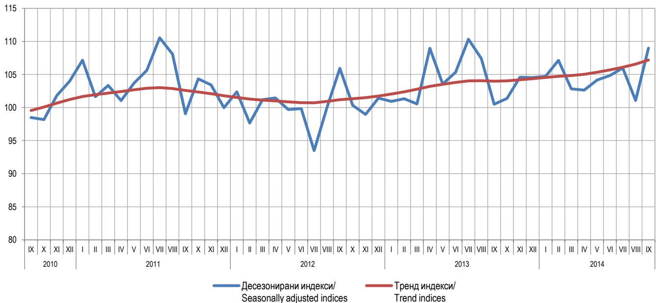
Графикон 1. Индекси индустријске производње, септембар 2010 – септембар 2014. (2010=100) Graph 1. Indices of industrial production, September 2010 – September 2014 (2010=100)
