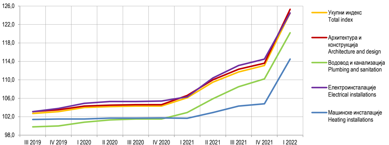
Графикон 1. Индекси произвођачких цијена у станоградњи Graph 1. Construction producer price indices for new residential buildings
