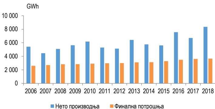
Графикон 16.1. Нето производња и финална потрошња електричне енергије
