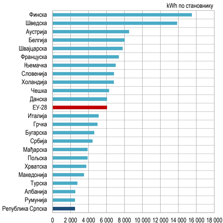
Графикон 16.2. Потрошња електричне енергије по становнику, 2013. (IEA)
